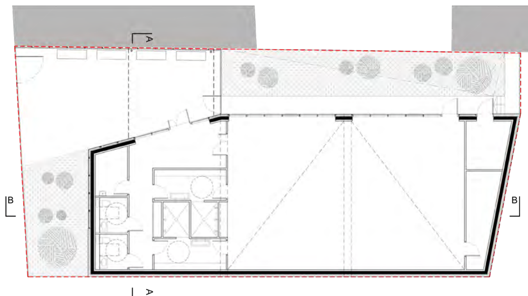
*Aménagement RDC
