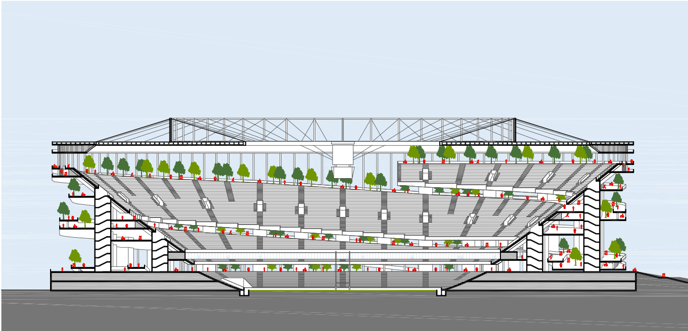
*coupe transversale
