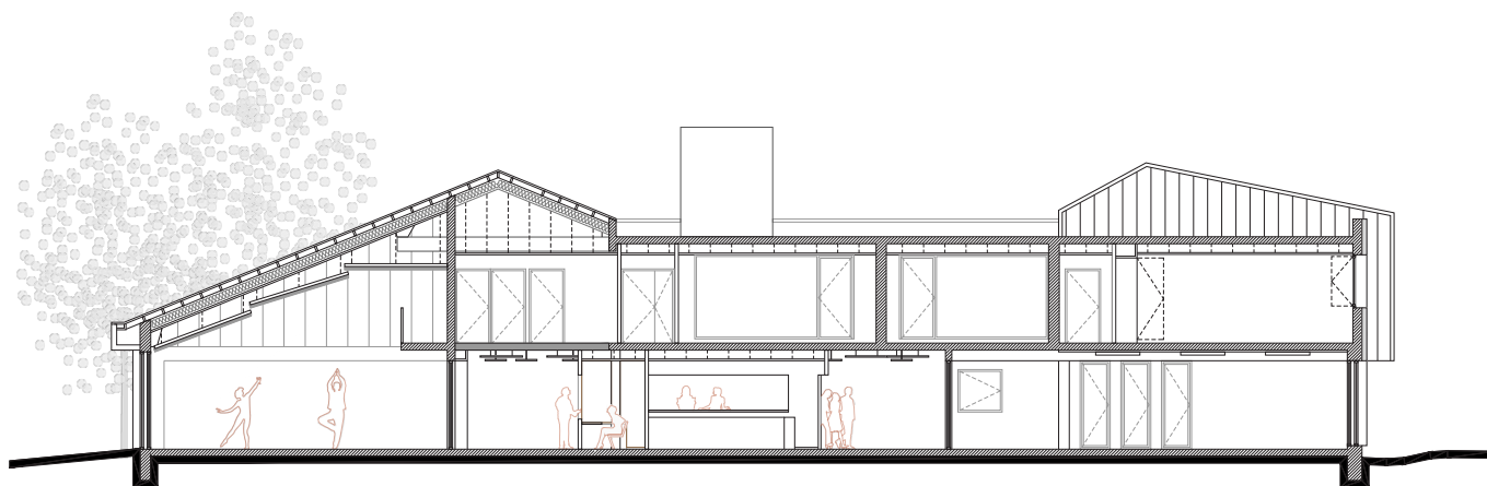
*Coupe longitudinale
