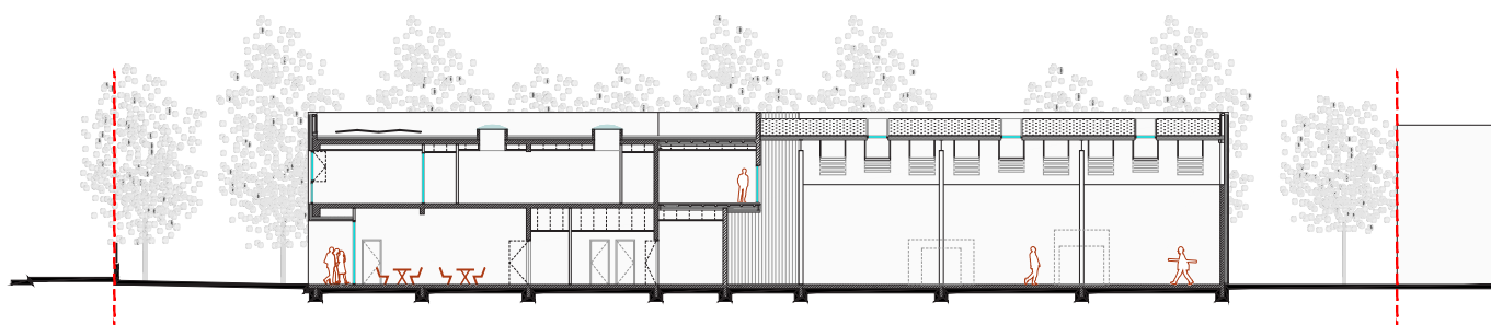
*Coupe longitudinale
